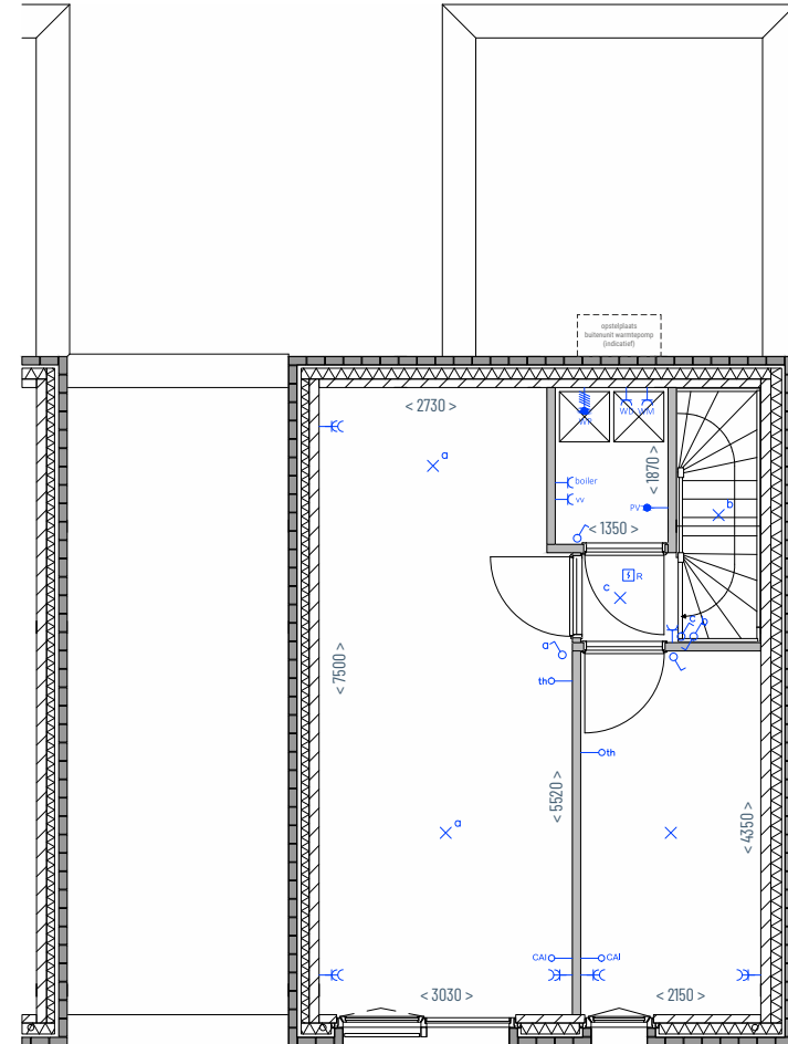
Technische tekening Woning A.02 Begane grond & eerste verdieping
